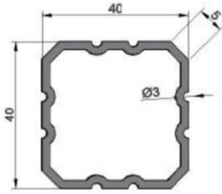
立柱
